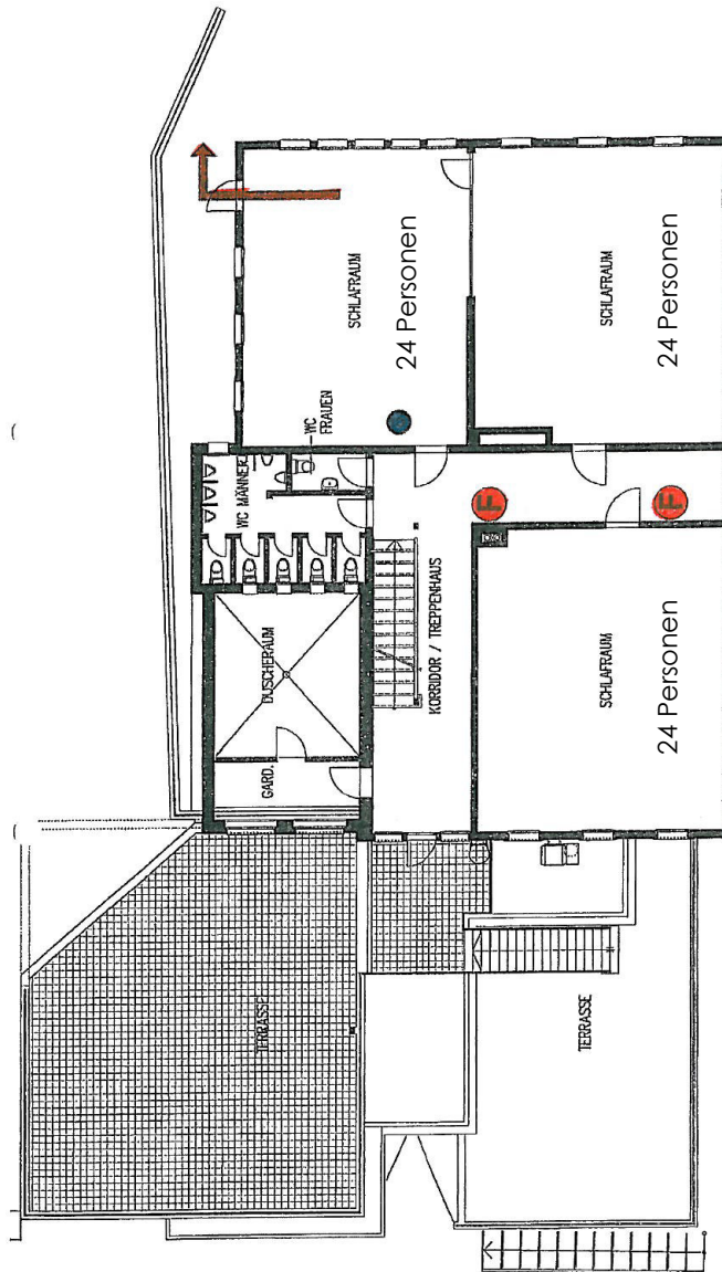
FLUCHTWEGPLAN Obergeschoss Ihr Standort Fluchtweg Wasserlöschposten od. Handfeuerlöcher
